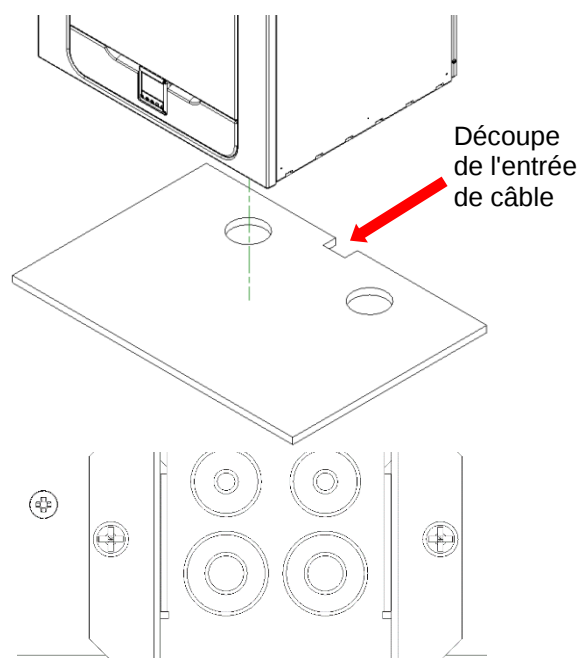
Entrée de câble du boîtier arrière
